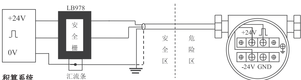
图（十一） 积算系统 LUGB/E B1 型
