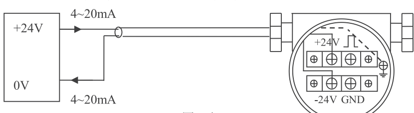
图（九） 积算系统
